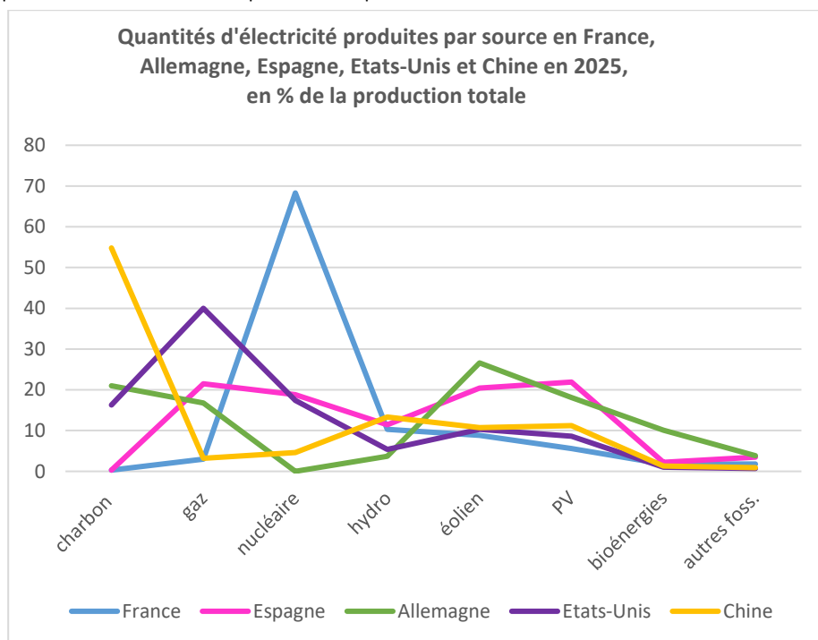
Figure 5- Quantités d'électricité produites par source en France, Allemagne, Espagne, Etats-Unis et Chine en pourcentage de leur production totale, d'après Ember's electricity data. A noter que la rubrique autres fossiles comprend ici le fuel et les déchets organiques. Ces derniers ne sont donc pas ici classés avec la bioénergie comme nous l'avons fait précédemment.
