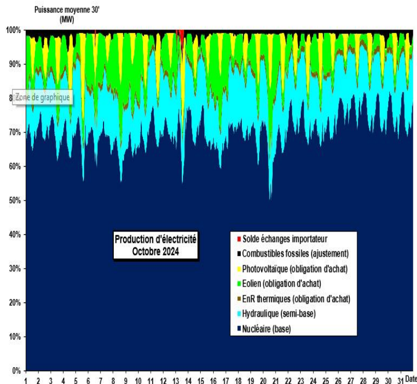
Figure 3 : Variations en Octobre 2024 des productions des différentes sources d'électricité en France, en % de la production totale. Données RTE, courtoisie JP Hulot. On constate que les pics de la production des non-pilotables, éolien et solaire PV, s'accompagnent d'une diminution importante de la part du nucléaire. Les pics de production fossile sont la conséquence de l'utilisation de TAC à fuel et à gaz pour faire face aux pointes de la consommation.
