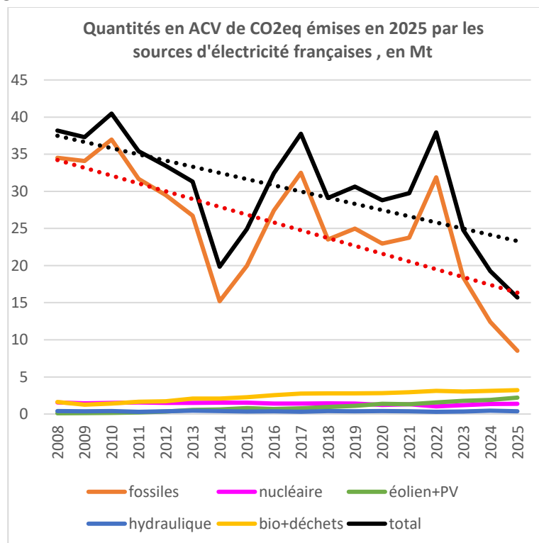
Figure 4 : Données ADEME et RTE. Quantités totales de CO 2 eq 2 , calculées en analyse de cycle de vie (ACV), émises par la production française d'électricité de 2008 à 2025, en millions de tonnes.
