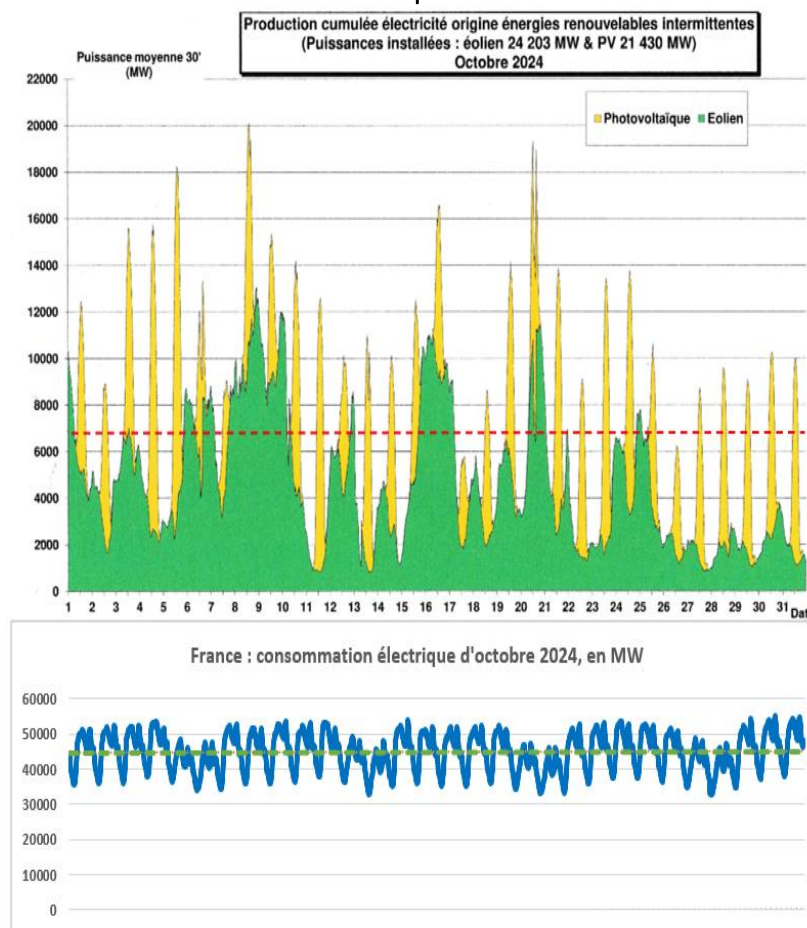
Figure 1 : Données RTE. Courtoisie JP Hulot. En haut : puissance délivrée en Octobre 2024 en France métropolitaine par l'ensemble des producteurs d'électricité éolienne (à terre et en mer) et d'électricité photovoltaïque. On observe la très grande variabilité de la puissance délivrée par l'éolien, avec de nombreux jours de puissance faible à très faible dus à l'absence quasi-totale de vent sur l'ensemble de la France, en particulier 5 jours de suite à la fin de ce mois. Les effondrements de la puissance délivrée, parfois jusqu'à quelques % de la
