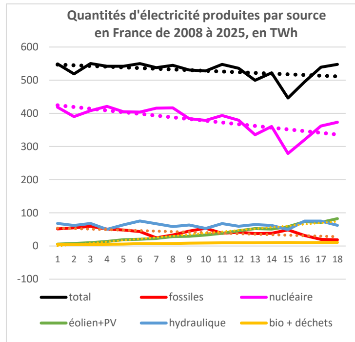
Figure 2 : Variations de 2008 à 2025 des quantités annuelles d'électricité produites par les différentes sources, en TWh. Données RTE. Suivant en cela les recommandations du Grenelle de l'environnement, la France a entre 2008 et 2025 progressivement et fortement augmenté ses capacités de production d'électricité éolien et solaire PV, sans pour autant augmenter sa production totale d'électricité. Celle-ci a même diminué.
